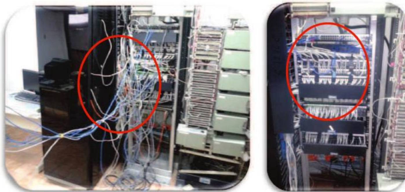
Reestructuración de cableado SITE de comunicaciones UTN (antes-después).
